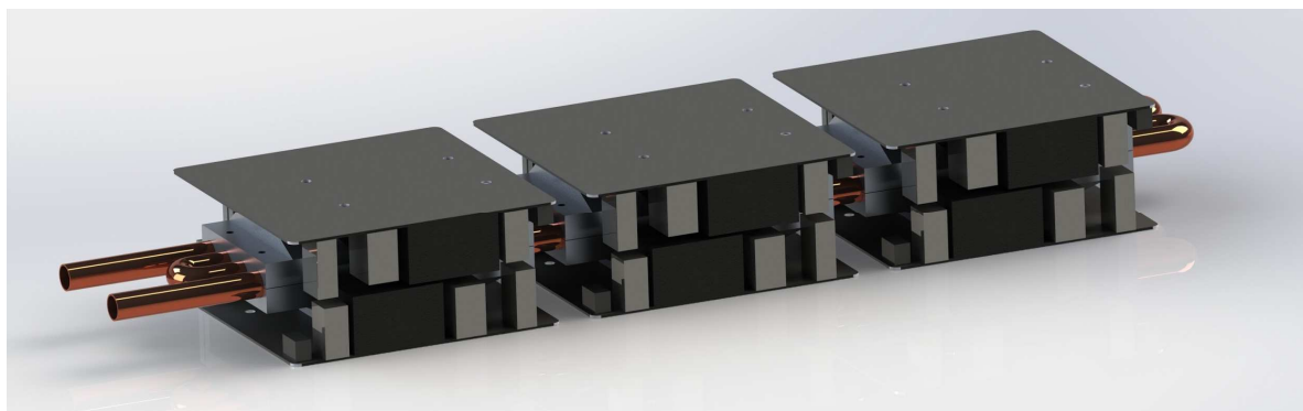
Figure 3 : Module de 6 carte mères de chauffage, jusqu'à 4 par chaudière numérique QB•1
