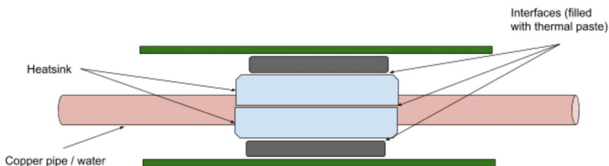
Figure 2 : Principe de chauffage ECS direct de la chaudière numérique QB•1
