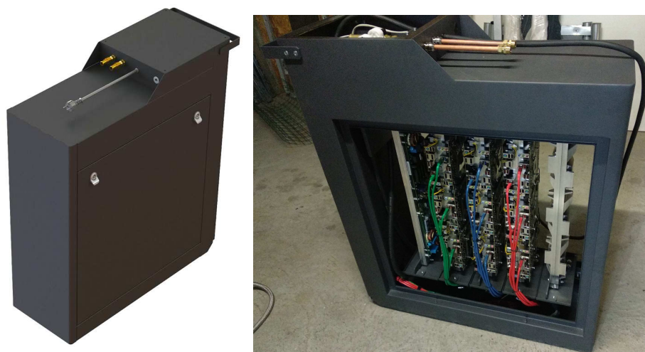
Figure 1 : Chaudière numérique QB•1
