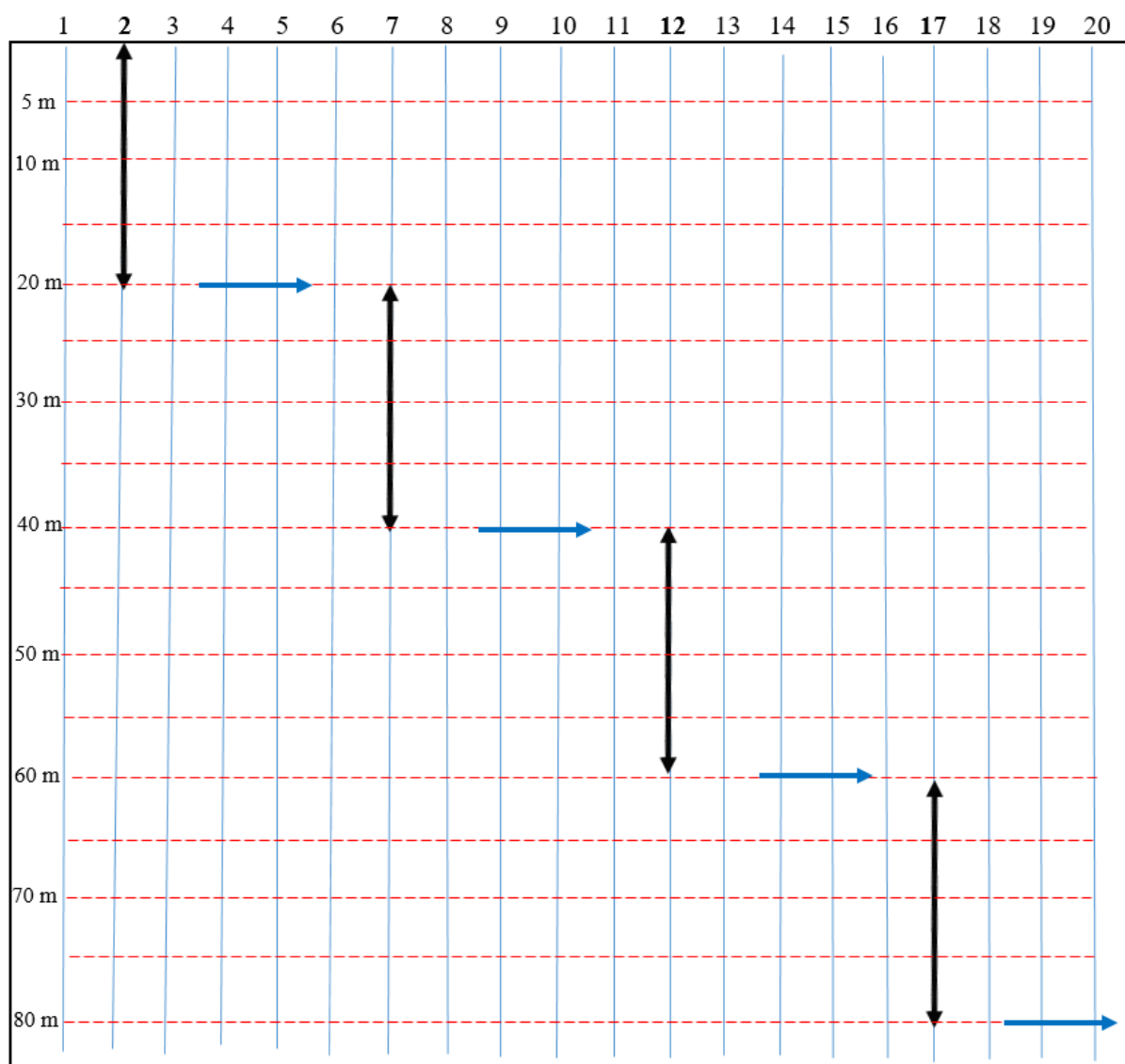
FIGURE 6. — Modèle d'échantillonnage pour la vérification d'un reboisement en feuillus réalisé par semis. Le déplacement se fait en « escalier » avec un comptage sur des échantillons de 20 mètres de long (traits en noir)
