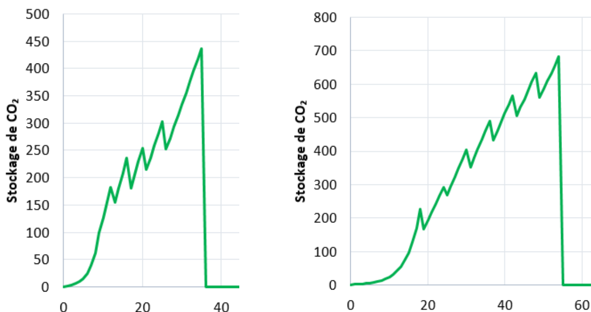
FIGURE 10. — Itinéraires sylvicoles du pin maritime (à gauche) et du douglas (à droite).
